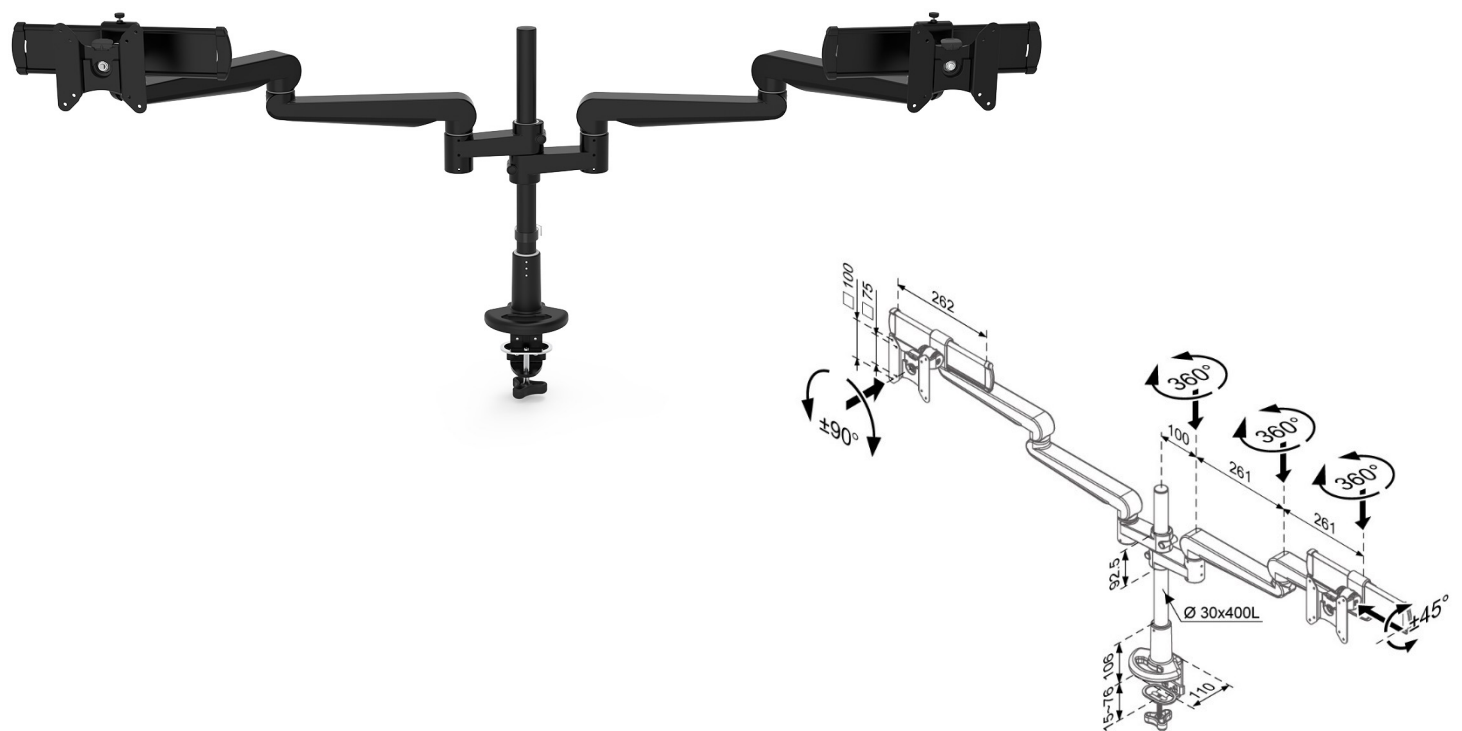
Clamp Type unit:mm
